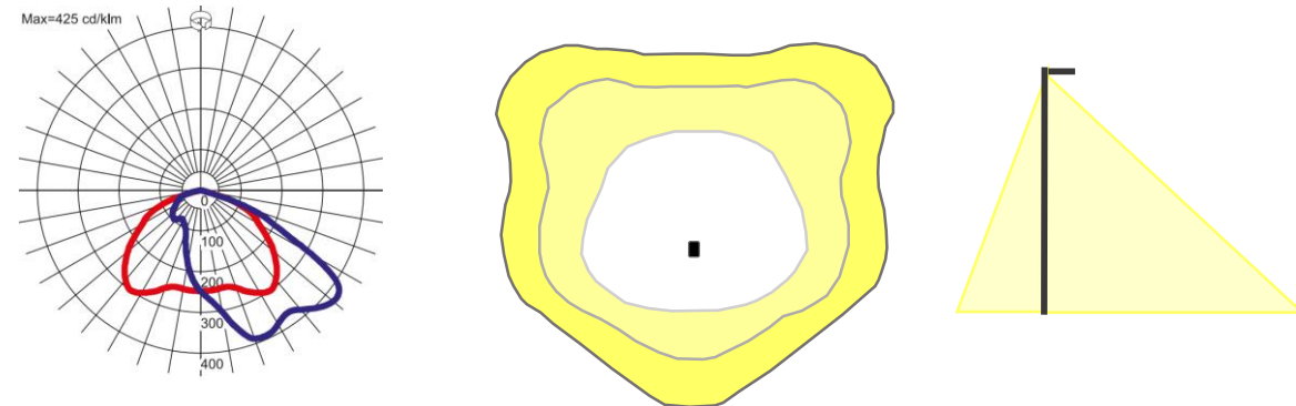
ACW – Assymetrisk bredstrålande strålkastaroptik
